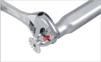
1. 安装喷淋头
